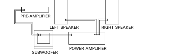
Conectar un par de cables de audio del enchufe de salida de preamp al enchufe de LINE IN de Subwoofer. Conectar el canal izquierdo a la izquierda y el canal derecho al derecho. Conectar un par de cables de audio de los enchufes de LINE OUT de subwoofer a los enchufes de entrada de amplificador. Conectar el canal izquierdo a la izquierda y el canal derecho al derecho.
